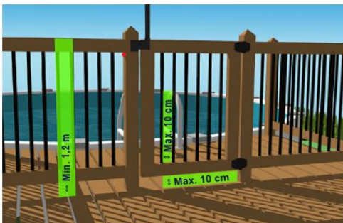
Dimensions exigées pour une enceinte.
