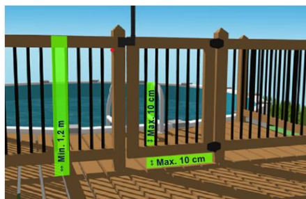
Dimensions exigées pour une enceinte.
