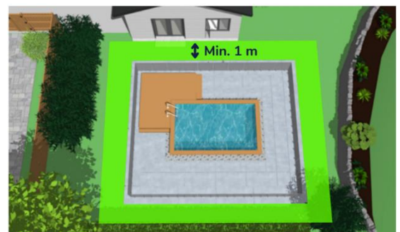
Exemple d'une enceinte de piscine située à plus de 1 m d'un mur de soutènement.
