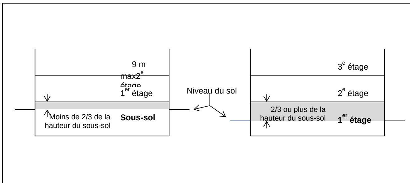
Figure 5 : Calcul demi-étage
